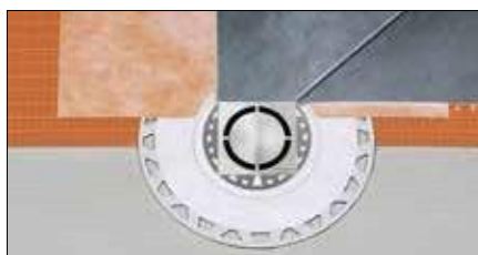
Schlüter® -KERDI-DRAIN Система підлогового слива для надійного підключення комбінованої ізоляції, створеною з допомогою Schlüter-KERDI , або інших герметизуючих систем до каналізації
