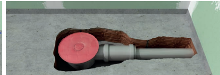
3. Приєднайте дренаж до вихідної труби, закрийте його отвір кришкою, перевірте нахил зливу
